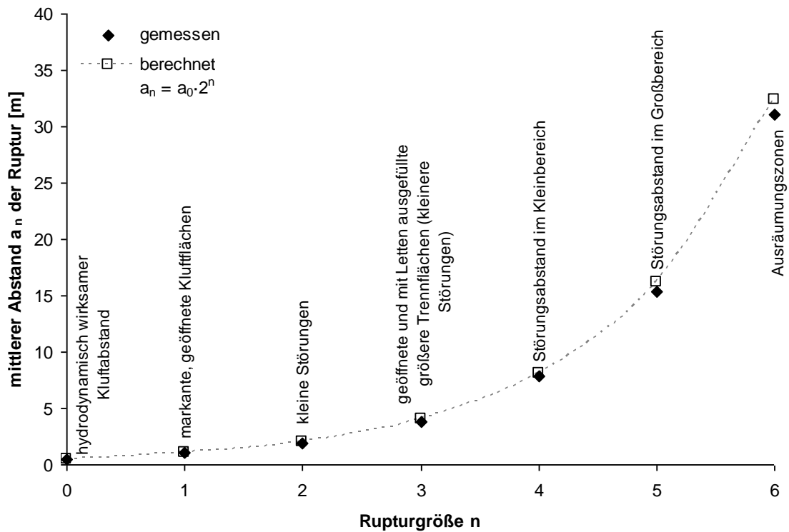
Abb. 6: Abhängigkeit des mittleren Rupturabstandes einer statistisch ermittelten Trennflächenschar (bc-Kluft) von der Rupturgröße (modifiziert nach MEIER 1978b)
