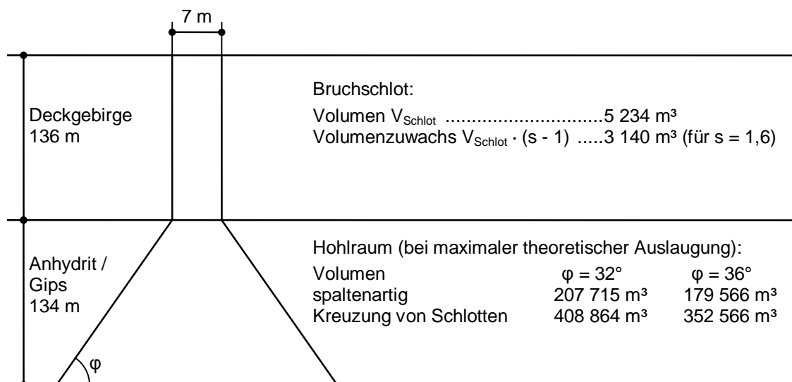
Abb. 10: Schematischer Schnitt durch den Erdfall auf der B 180 mit maximalen Hohlraum-Bruchvolumen-Bilanzen
