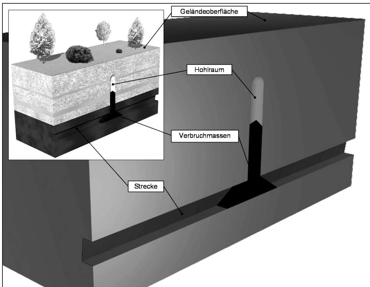
Abb. 2: Schematisches Blockbild eines Hochbruches über einer Strecke
